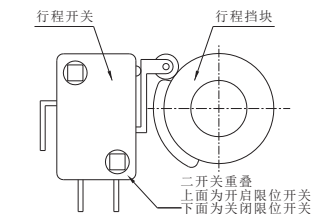
CX-05/15行程挡块和行程开关布局图
