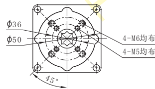
直装式外形尺寸
