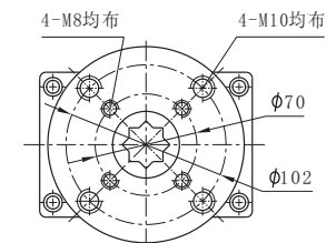
直装式外形尺寸
