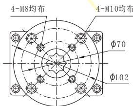
直装式外形尺寸
