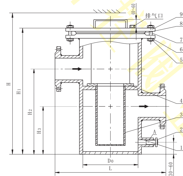
TGG 结构图
