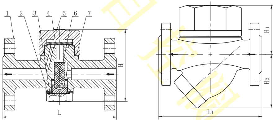
CS49系列T型结构图
