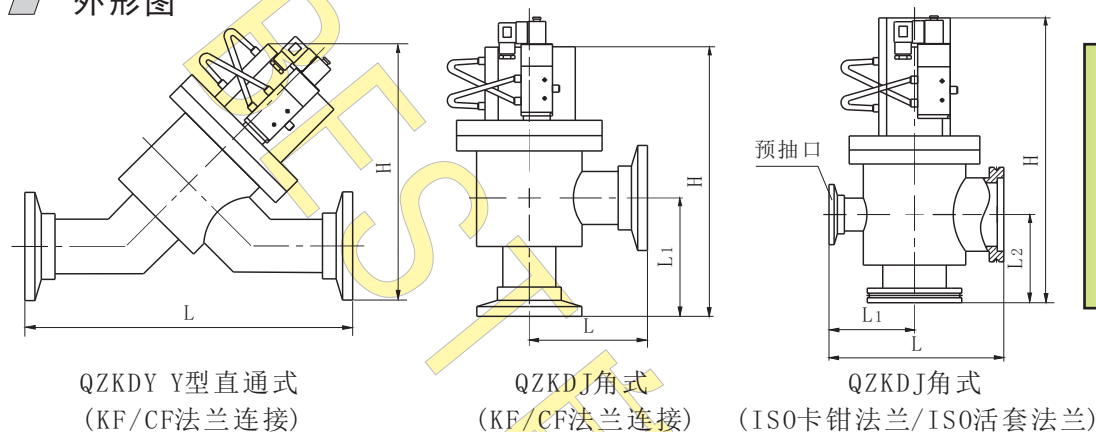
QZKDJ-50B[CF]Ib24 (CF法兰连接)
