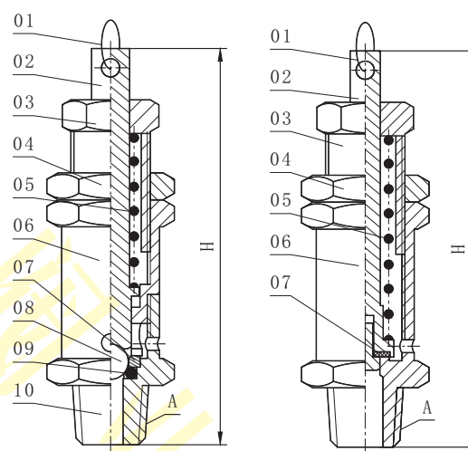
DN06~10结构图
