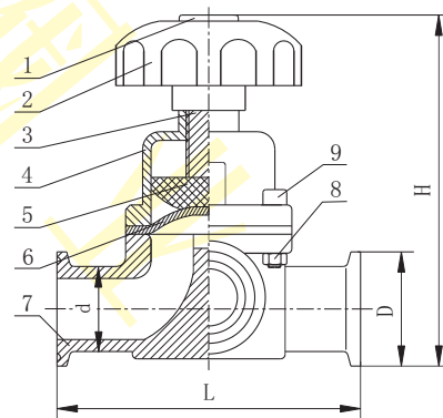
卡箍连接
