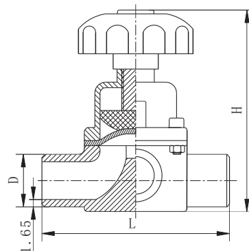
对焊连接
