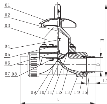
承插焊连接
