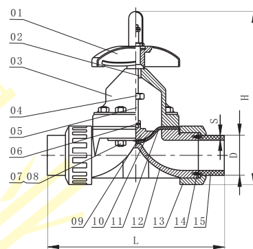
对焊连接
