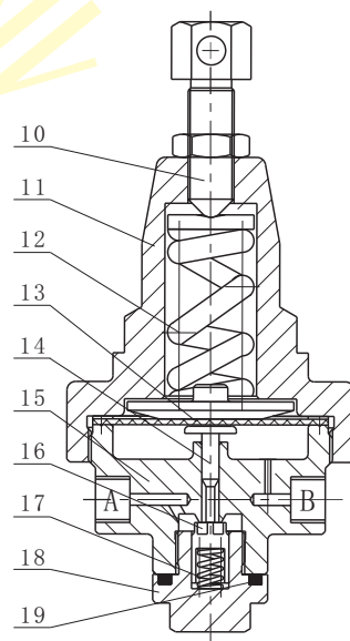
导阀结构图
