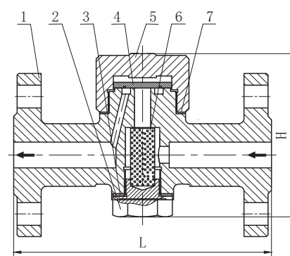
CS49系列T型结构图
