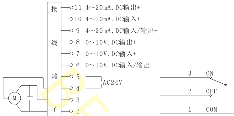
智能调节型控制线路图
